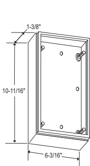
1 1/2" Conduit Adapter Back Box (CA)
